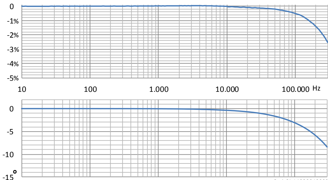
Gain/Phase
